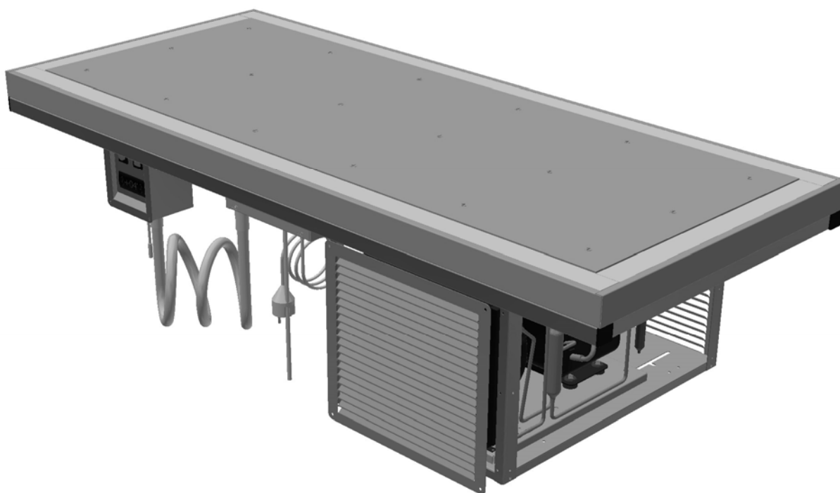
Kjøleplate for undermontering uten stativ RBKP-UM, se side 88
